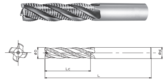
HSS-Co 単位:mm Unit:mm
